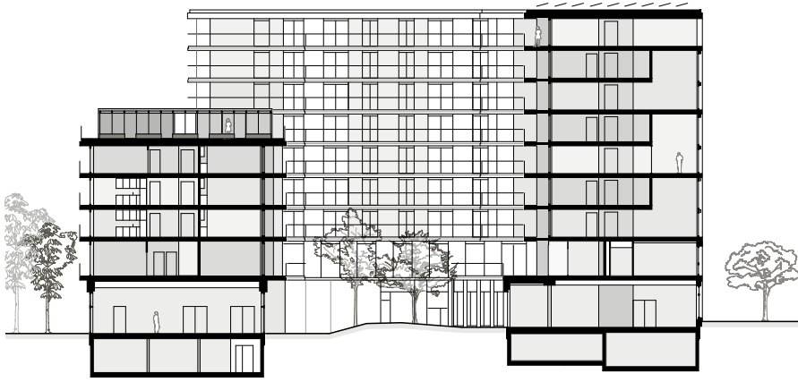
Coupe transversale · Querschnitt
